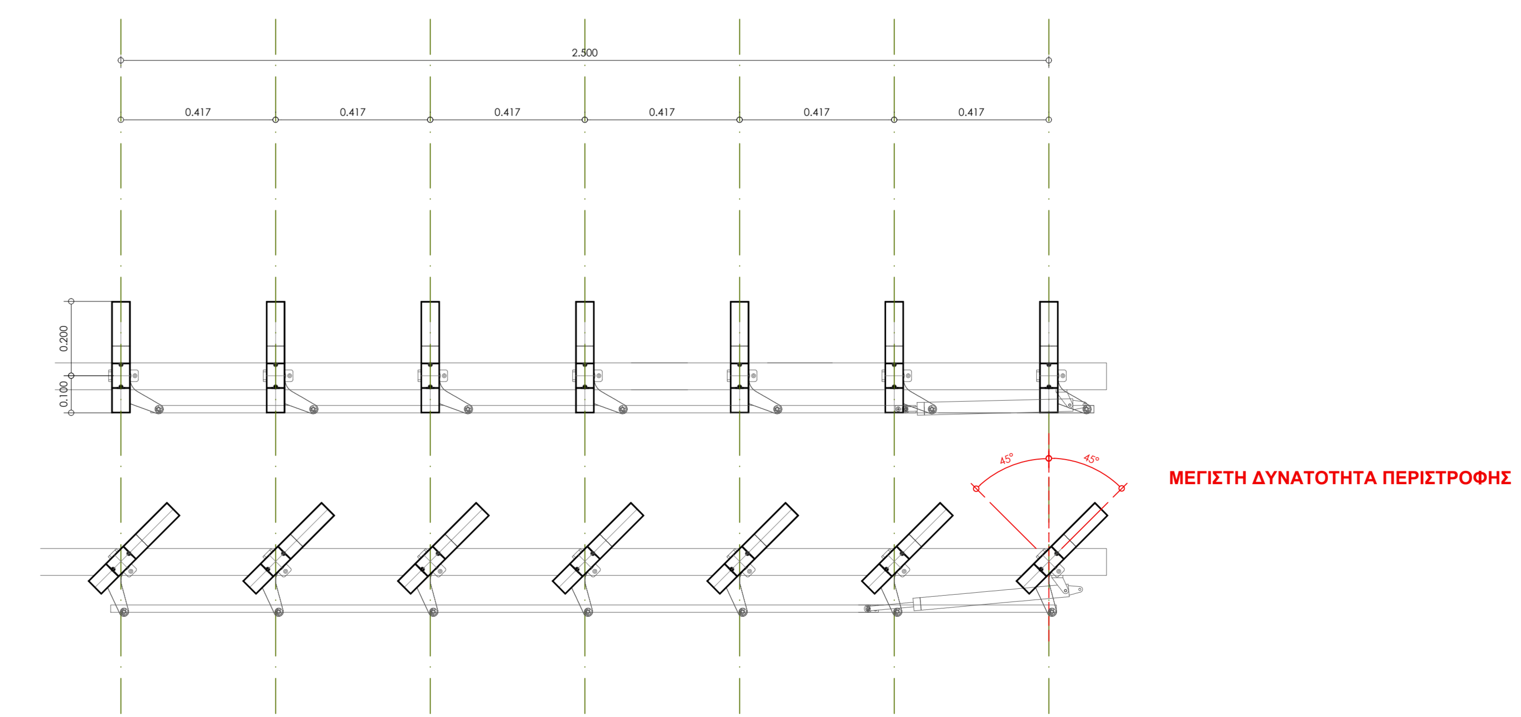
1/10 _ ΚΑΤΟΨΗ ΣΥΣΤΗΜΑΤΟΣ ΠΕΡΣΙΔΩΝ
