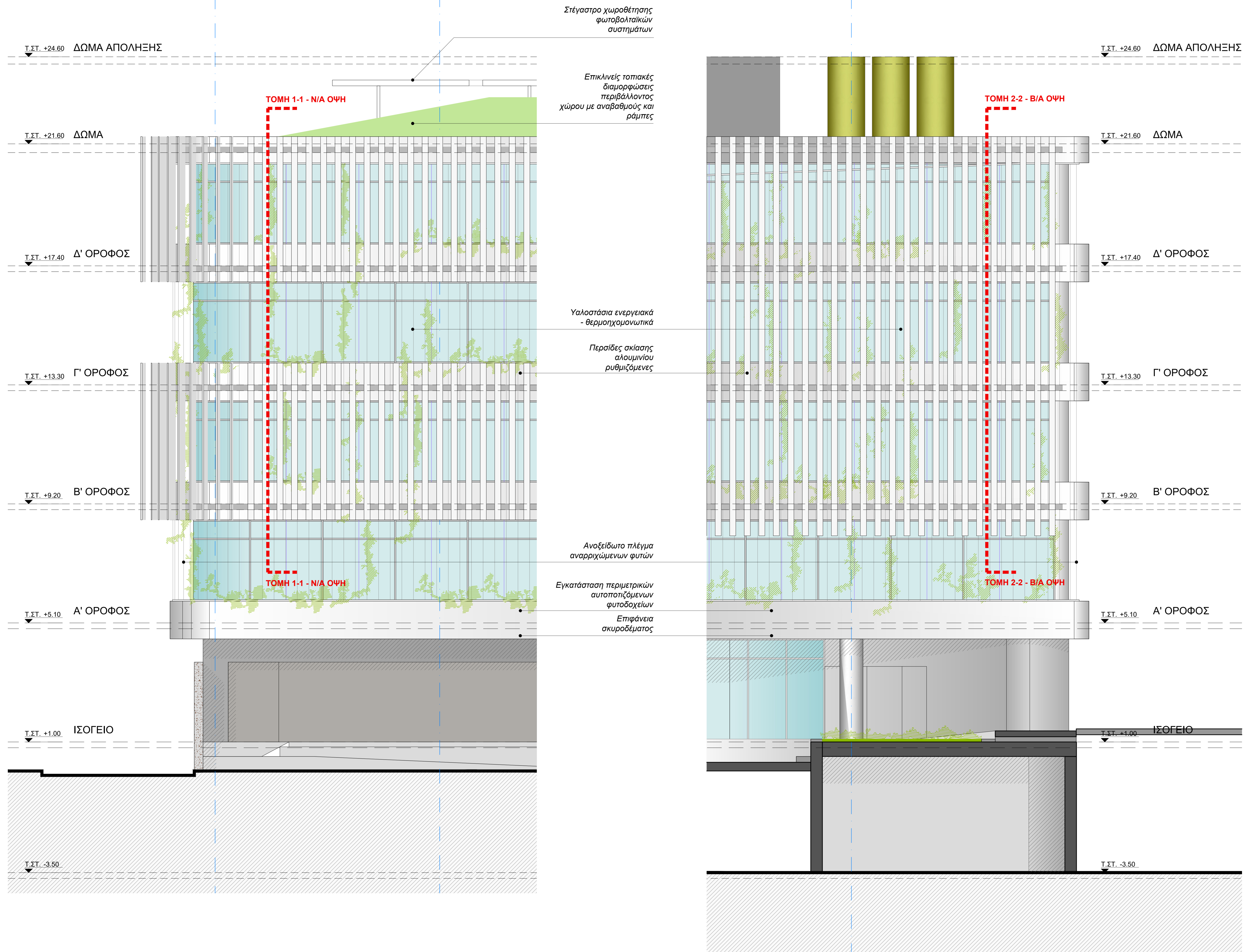
1/50 _ ΤΜΗΜΑ Ν/Α ΟΨΗΣ
