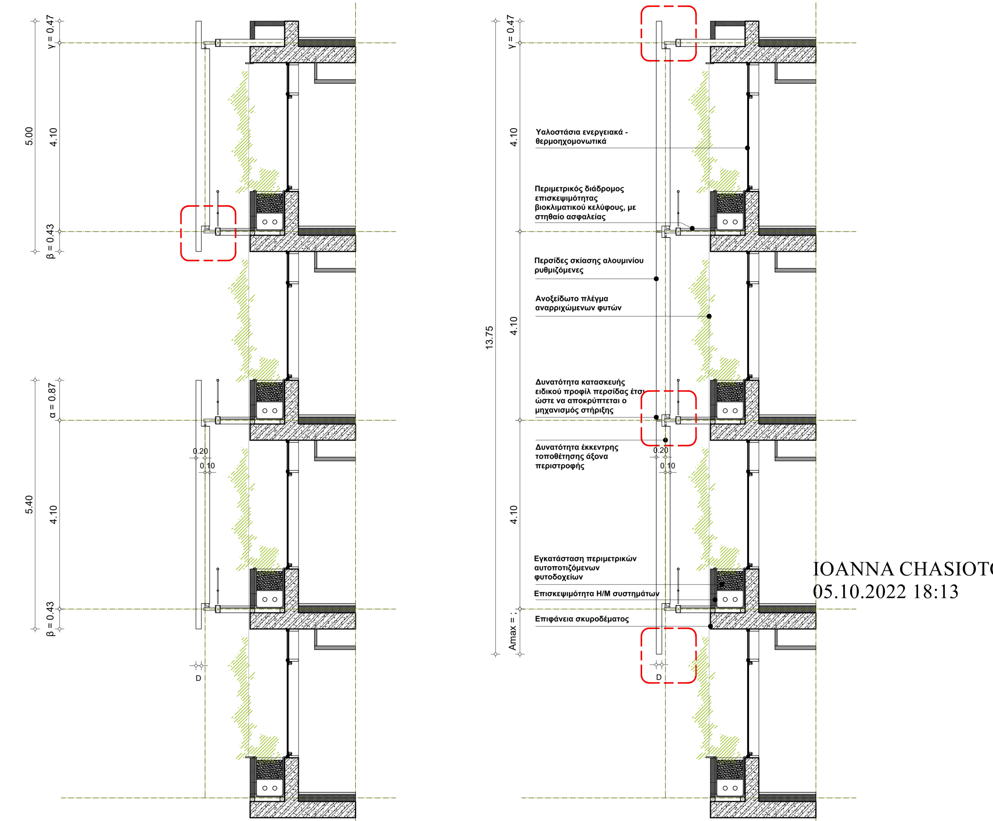
ΤΟΜΗ 1-1 - Ν/Α ΟΨΗ
